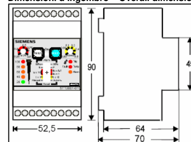
Dimensioni d'ingombro - Overall dimension - Dimensiones (mm)
