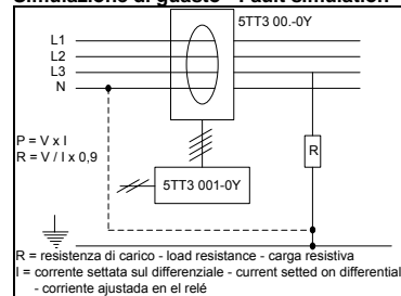
Simulazione di guasto - Fault simulation - Simulación de defecto
