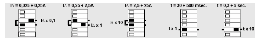
Scelta della gamma di taratura della corrente e del ritardo - Setting the current tripping range and delay - Ajuste del rango de la sensibilidad y del tiempo de retardo
